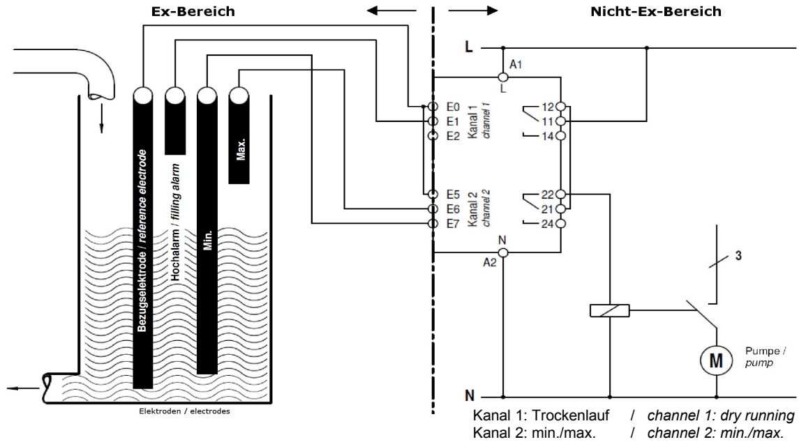
Ruhestrom: Behälter füllen / closed circuit current: fill the container
