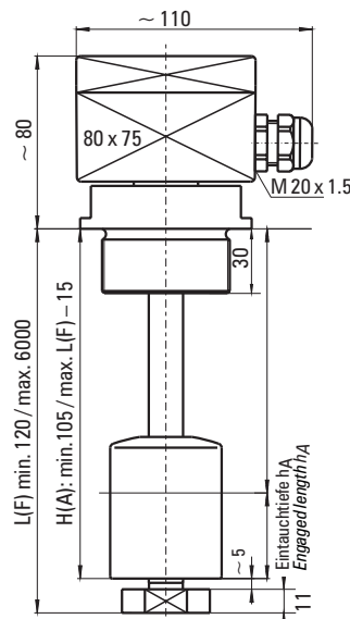
Maßbild 2: feste Ausführung mit G 2¼" und Dose Dimensioning figure 2: Fixed version with G 2¼" and connector box
