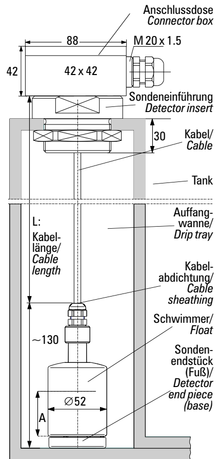
Leckagesonde mit standsicherem Fuß, auf dem Boden aufstehend Leak detector with firm base, floor mounted
