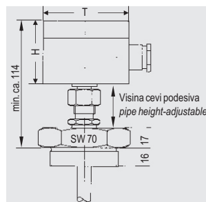
Tip / Type RMS-VMS-A2"-AA(PO)-V } = obezbedjeno RVA-VMS-A2"-AA(PO)-V } spojem cevi RMS-VVA-A2"-AA(PO)-V } Secured with RVA-VVA-A2"-AA(PO)-V } tube union
